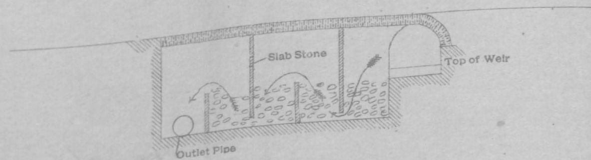
SECTION ON A. A.
