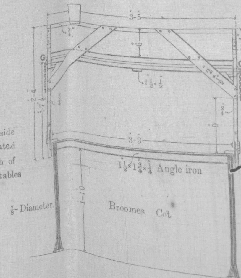
DETAILS OF TABLE PIVOT AT G. G.
