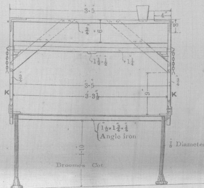
DETAILS OF W IRON BRACKETS AT K. K.
