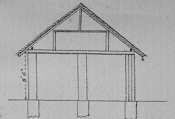
SECTION A.B.
