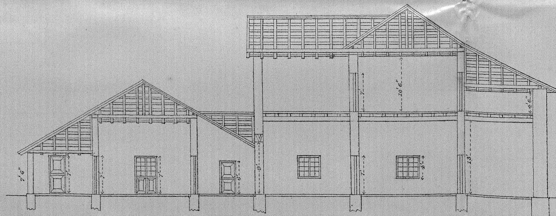
SECTION A.B.
