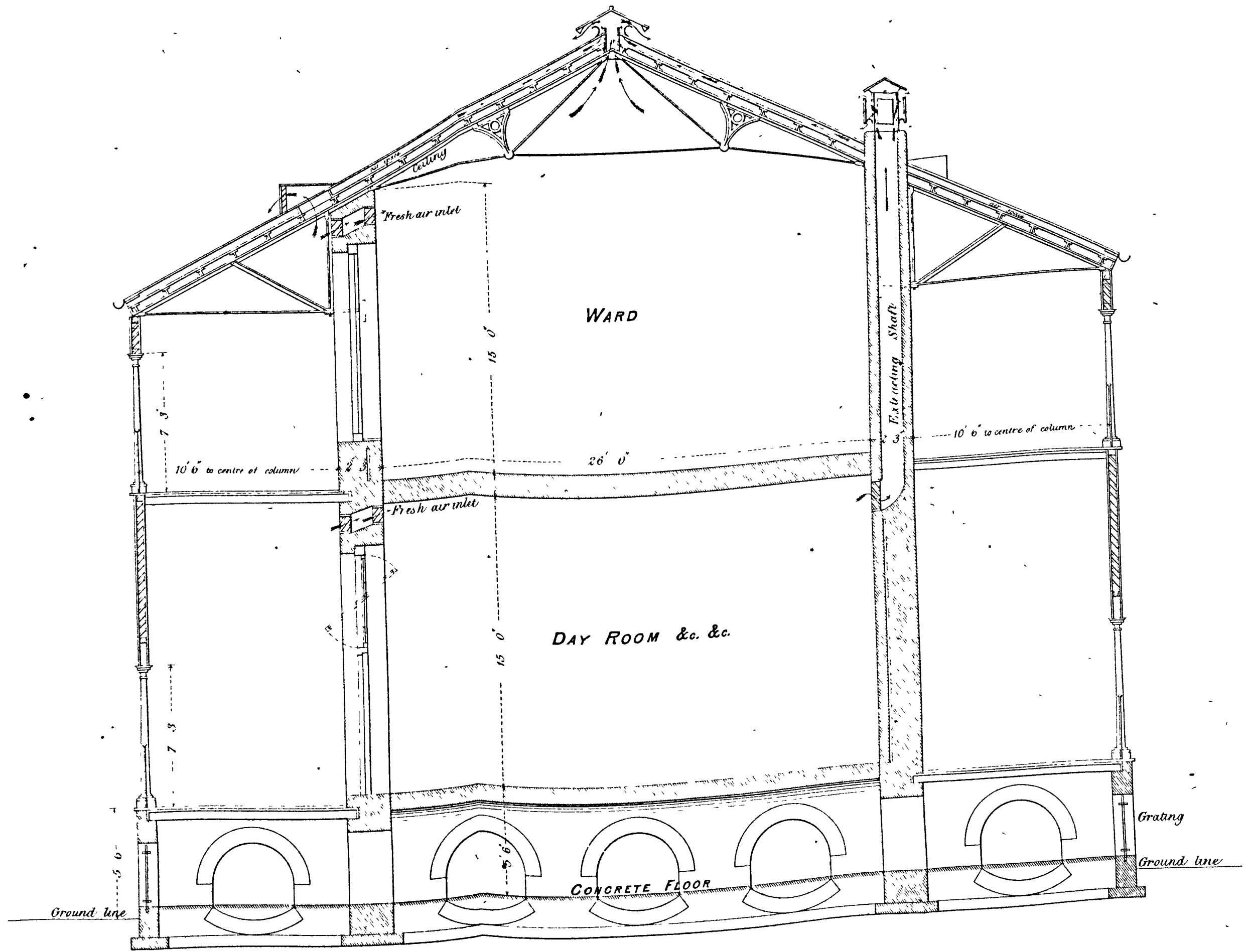
SECTION A.B.
