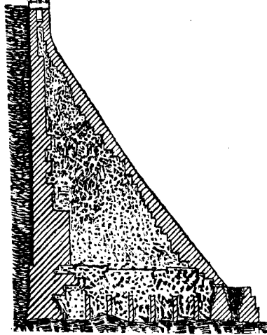
அணைகளின் குறுக்குவெட்டுப் பார்வை.
