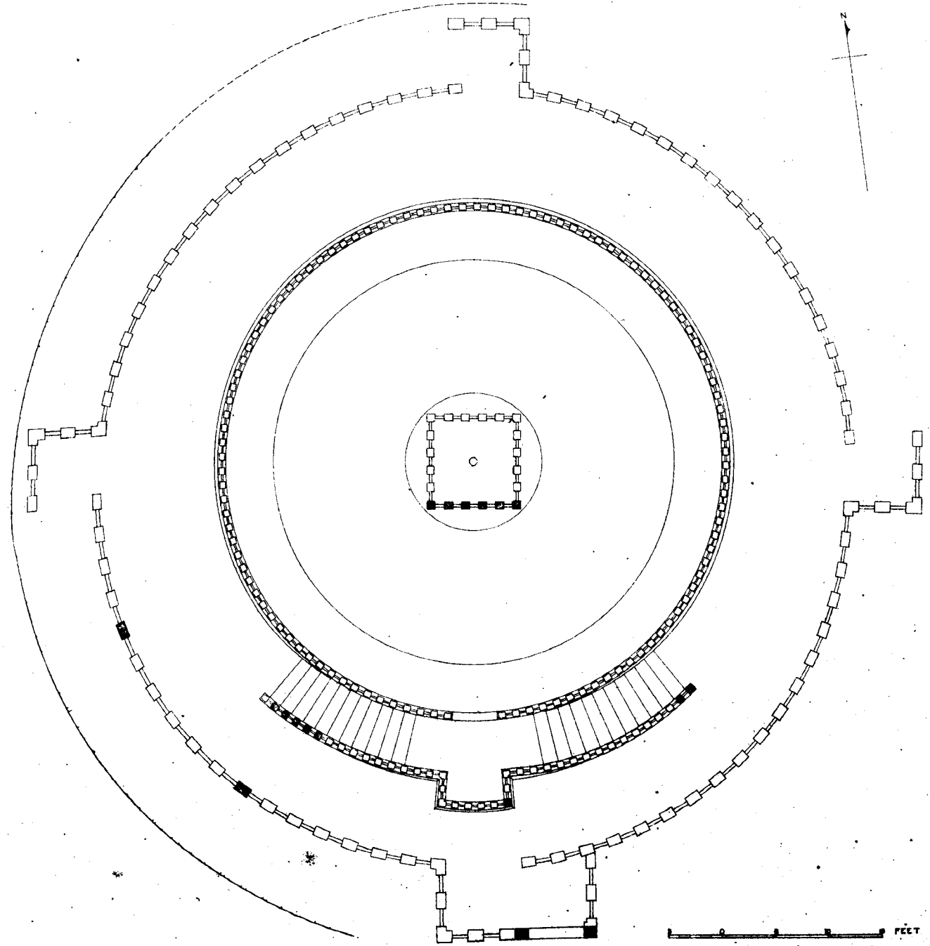
b. PLAN.
