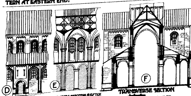
PART EXTERIOR ELEVATION (D) PART LONGITUDINAL SECTION (E)
