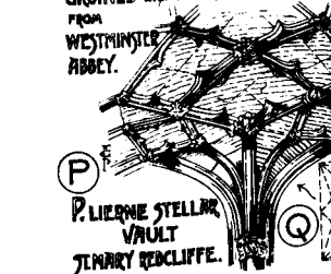
P. LIERNE STELLAR VAULT.
