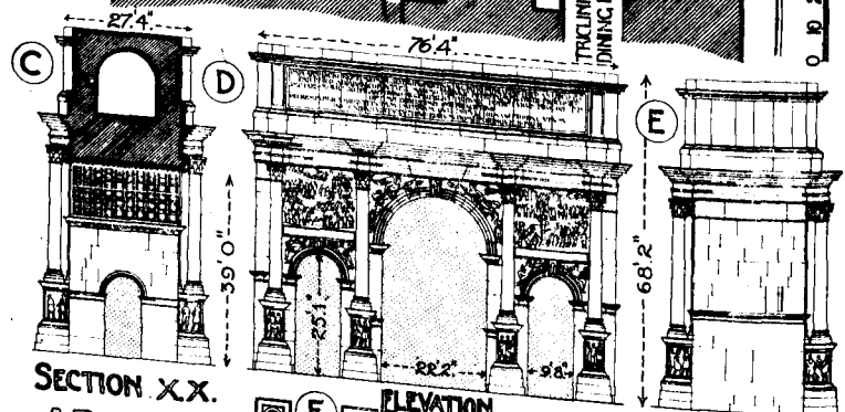
END ELEVATION
