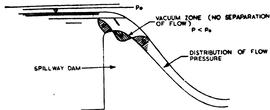
FIG. 1 SPILLWAY DAMS
