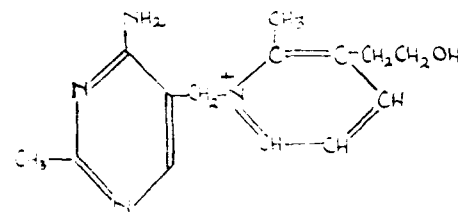
Pyriethamine.
