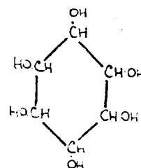
Inositol.
