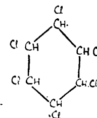
Gammaxane.
