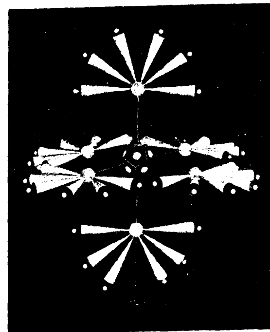
FIG. 19. BENZENE C_6H_6
