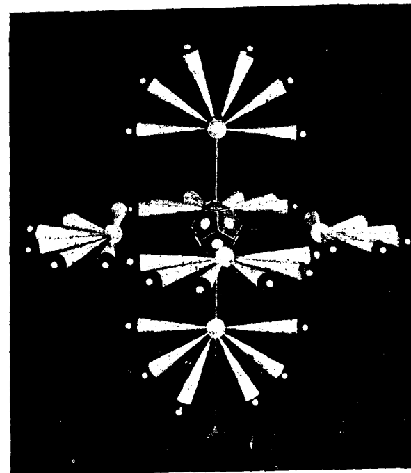
FIG. 18. BENZENE C_6H_6
