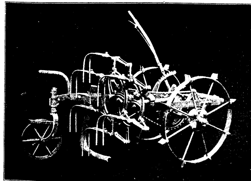
FIG. 1. Improved Potato Digger (Link Type).
