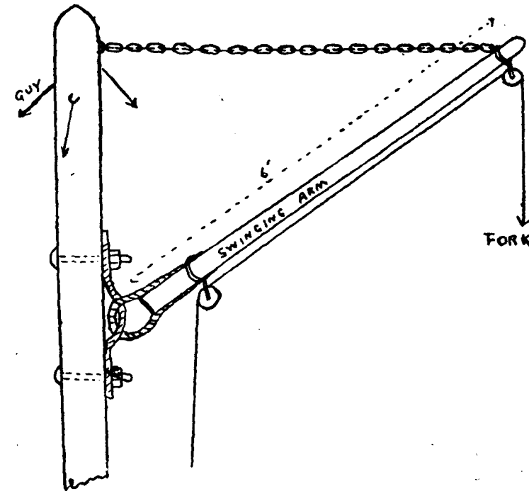
FIG. 3.—A Simple Jib.
