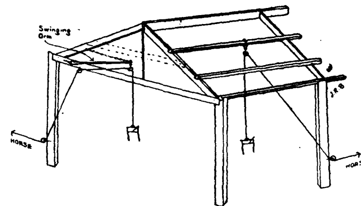
FIG. 4.—Barn Forks.
