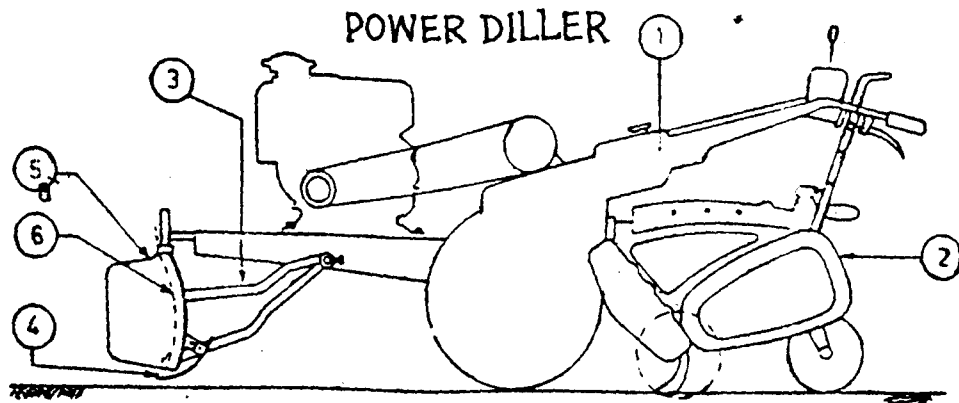
பவர்டில்லரால் இயங்கும் சமப்படுத்தும் - வரப்பு அமைக்கும் கருவி
