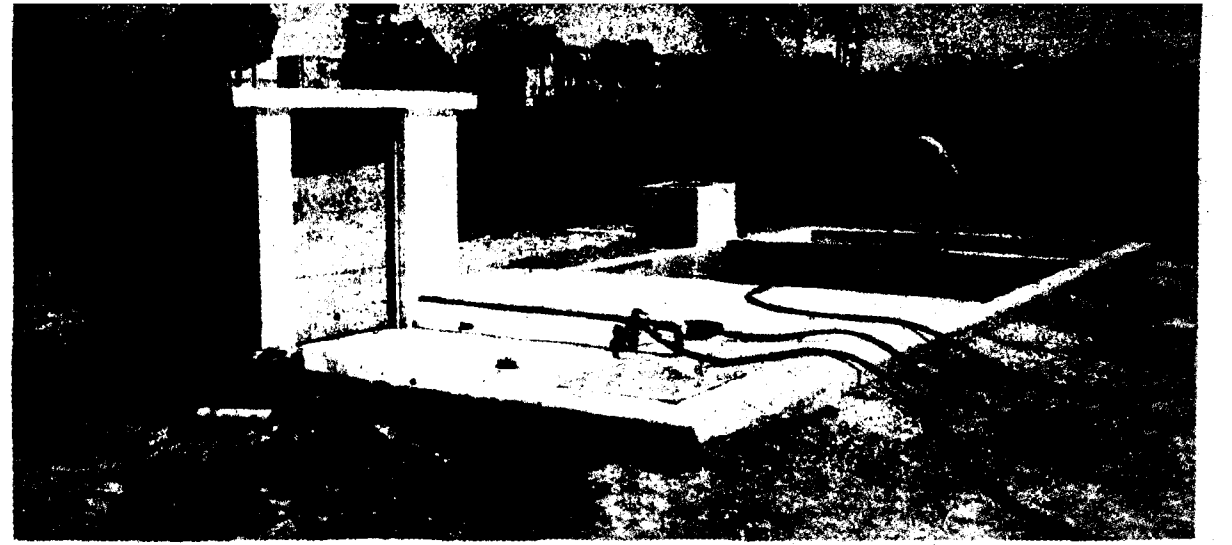
நீரைக் காய்ச்சி பன்னீர் வடித்தெடுக்கப் பயன்படும் சூரிய வெப்பத்தால் இயங்கும் கருவி.
