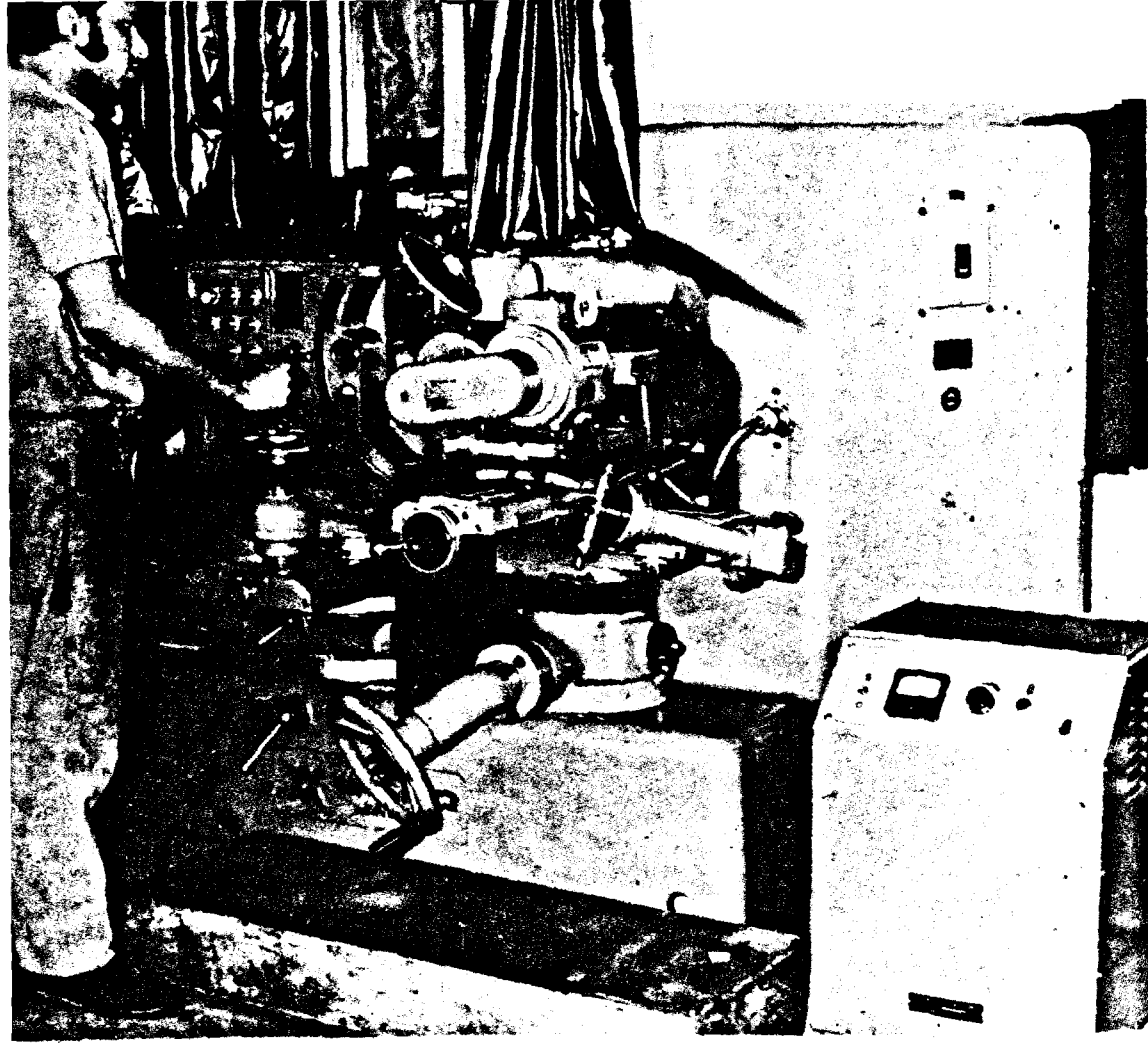
‘சிப்பெட்’ பயிற்சி நிலையத்தில் நவீன இயந்திரங்களைக் கொண்டு பிளாஸ்டிக் தொழிலில் கல்வியளிப்பதில் அளிக்கப்படுகிறது.
