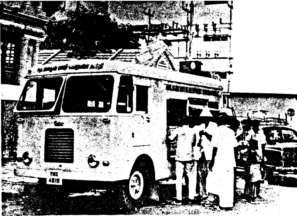
நடமாடும் பால் விற்பனை ஊர்தி.
