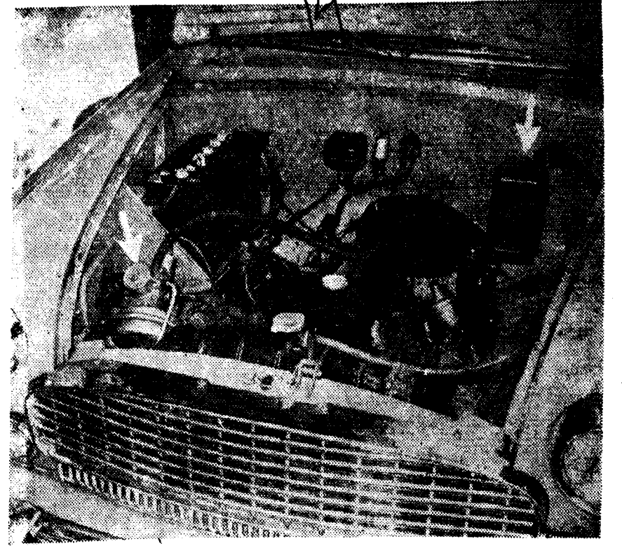
அமெரிக்காவில் பயிற்சி பெற்ற தமிழ் நாட்டுப் பொறியியலர் கண்டுபிடித்த மின் சக்தியாக இயங்கும் 'ஷ்பூர் ஸ்டாப்' எனப்படும் பிரேக்கும் (இடதுபுறம் உள்ளது) இயந்திரத்தைக் குளிரவைக்கும் 'நியோகூல்' பகுதியும் (வலதுபுறம் உள்ளது) படத்தில் அமைந்திருப்பதை காணலாம்.
