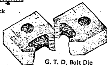
G. T. D. Bolt Die
