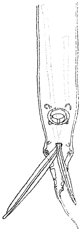
Fig. 55.— Heterakis isolonche . Posterior end of male; ventral view. (After Lucet and Henry.)
