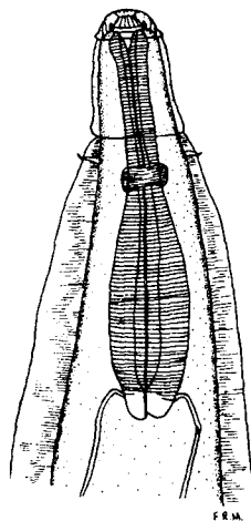
Fig. 136.— Esophagostomum columbianum . Anterior end; dorsal view. (From Baylis, after Ransom.)
