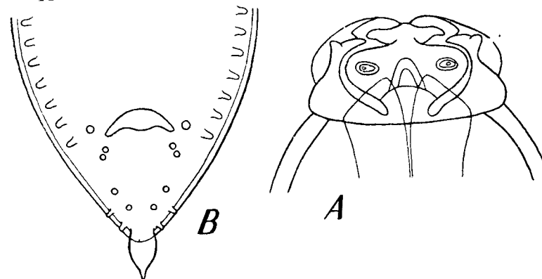
Fig. 35.— Contracæcum tricuspe . A, head, dorsal view; B, posterior end of male, ventral view. (After Gedoelst.)
