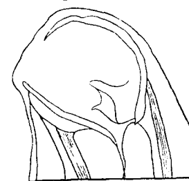
Fig. 150.— Globocephalus connorfilii . Anterior end; lateral view. (After Lane.)
