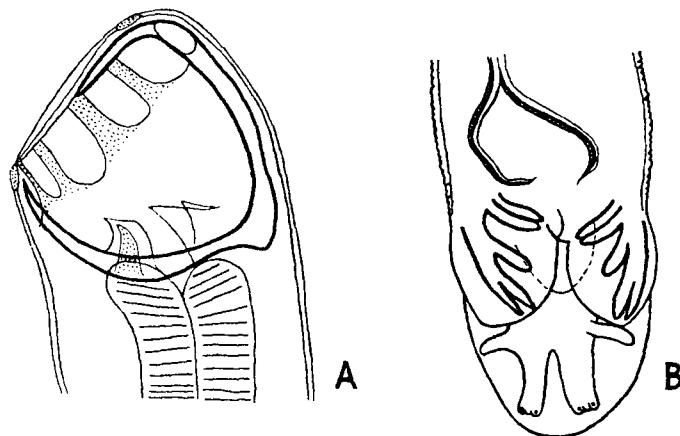
Fig. 154.— Gaigeria pachyseclis . A, anterior end, lateral view; B, posterior end of male, ventral view. (After Yorke and Maplestone.)
