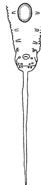
Fig. 79.— Kathlania chiloscyllyi . Anterior end; dorsal view. (After Thwaite.)
