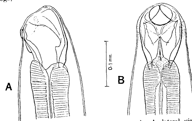
Fig. 155.— Uncinaria stenocephala . Anterior end. A, lateral view; B, dorsal view. (After Baylis, in 'Parasitology'.)
