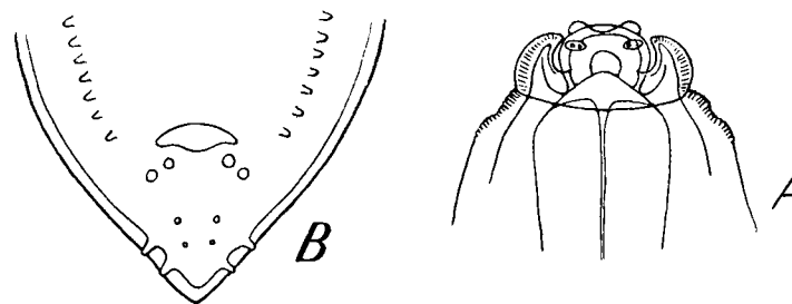
Fig. 33.— Contracæcum microcephalum . A, head, dorsal view; B, posterior end of male, ventral view. (After Geddoelst.)
