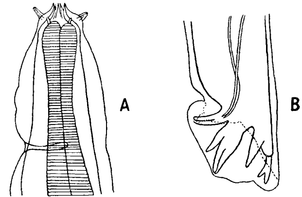
Fig. 135.— Æsophagostomum dentatum . A, anterior end, lateral view; B, posterior end of male, lateral view. (After Yorke and Maplestone.)
