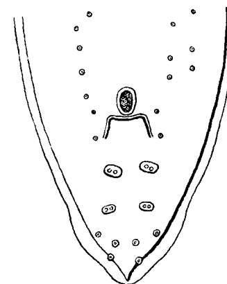
Fig. 2.— Ascaris lumbricoides . Posterior end of male; ventral view. (After Schneider.)
