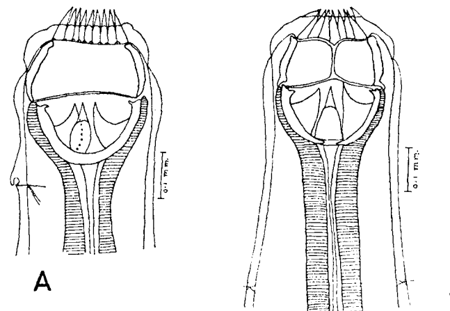
Fig. 140.— Æsophagostomum tridentatum . Anterior end. A, lateral view; B, dorsal view. (After Maplestone.)
