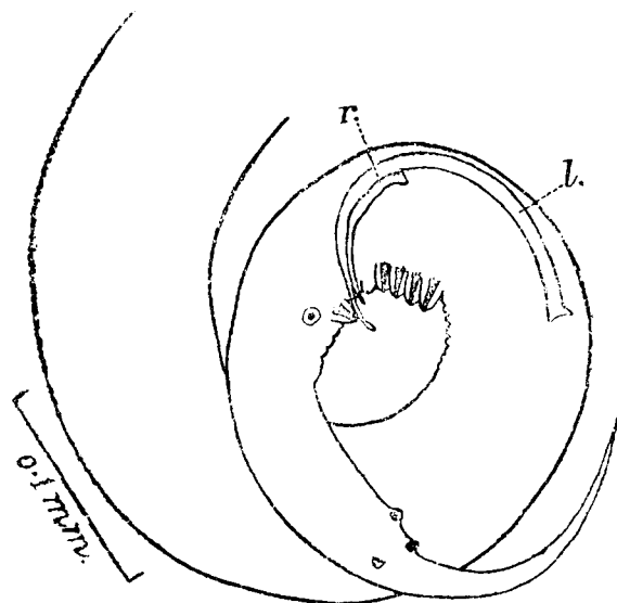
Fig. 110.— Monhysterides piscicola . Posterior end of male; lateral view. l. , left spicule; r. , right spicule. (After Baylis and Daubney.)
