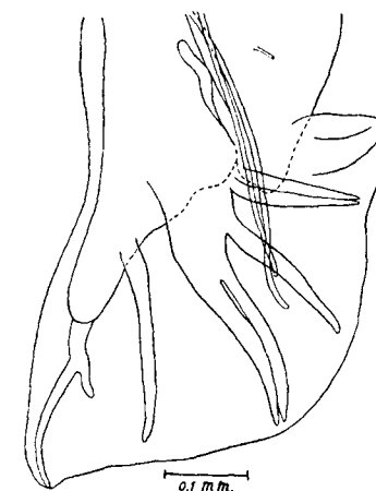
Fig. 138.— Æsophagostomum blanchardi . Anterior end. (After Travassos and Vogelsang.)
