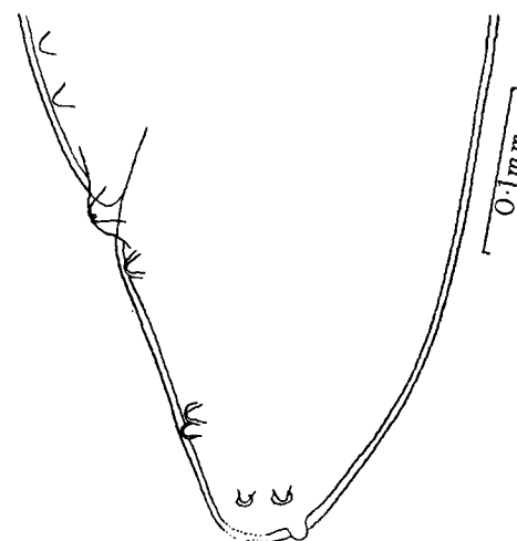
Fig. 17.— Polydelphis rotundicaudata . Posterior end of male; lateral view. (Original.)
