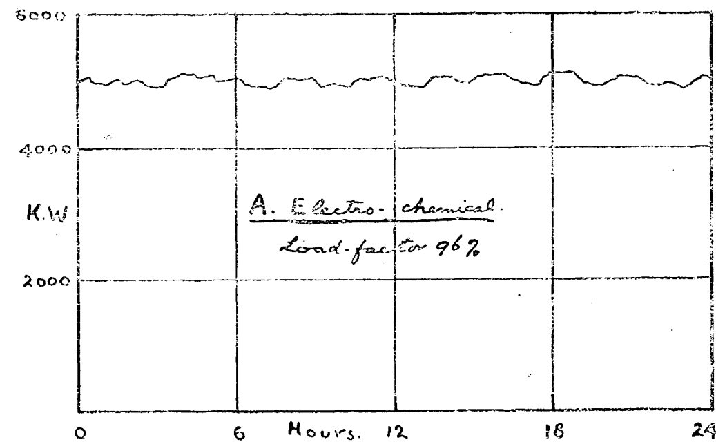
Fig. 16. Load factor diagram.
