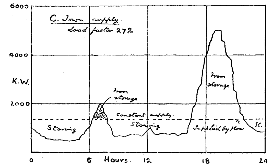
Fig. 18. Load factor diagram.
