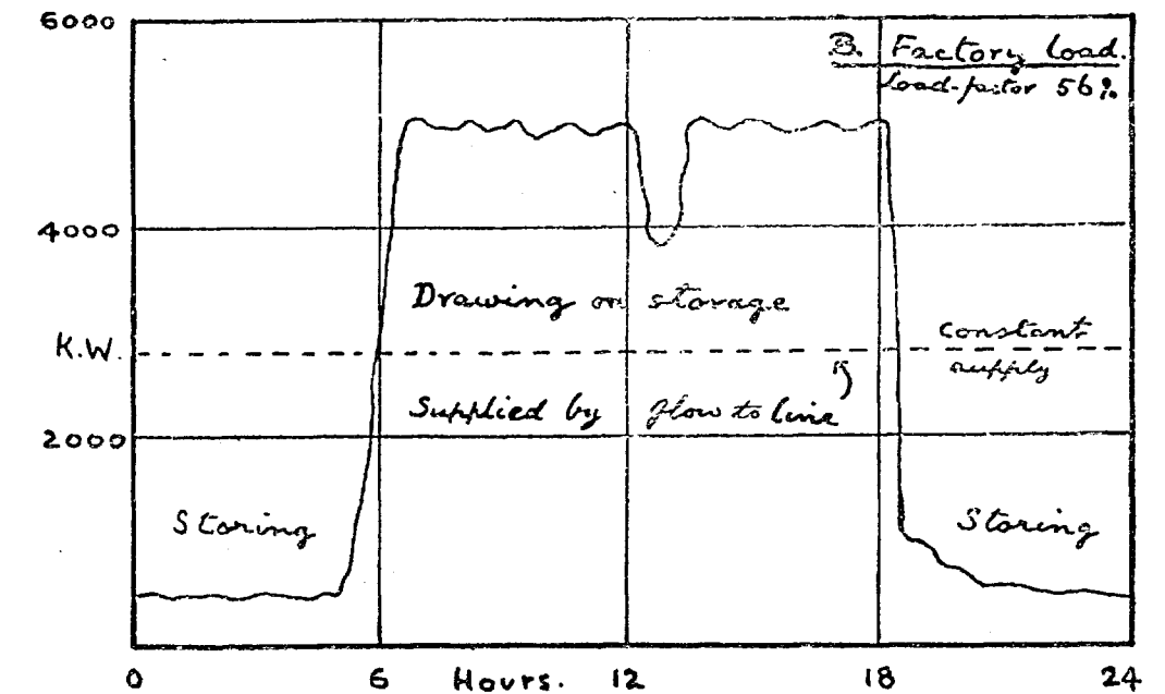
Fig. 17. Load factor diagram.
