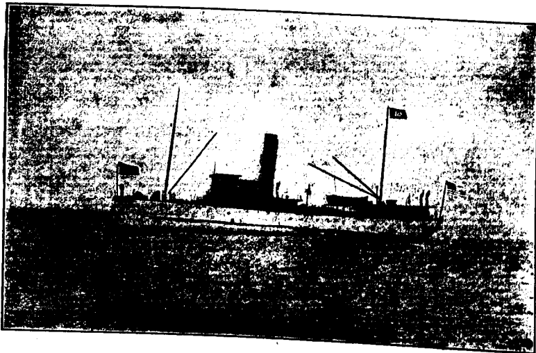
FIG. 55.—U. S. Sea-going Dredge "Burton,"
