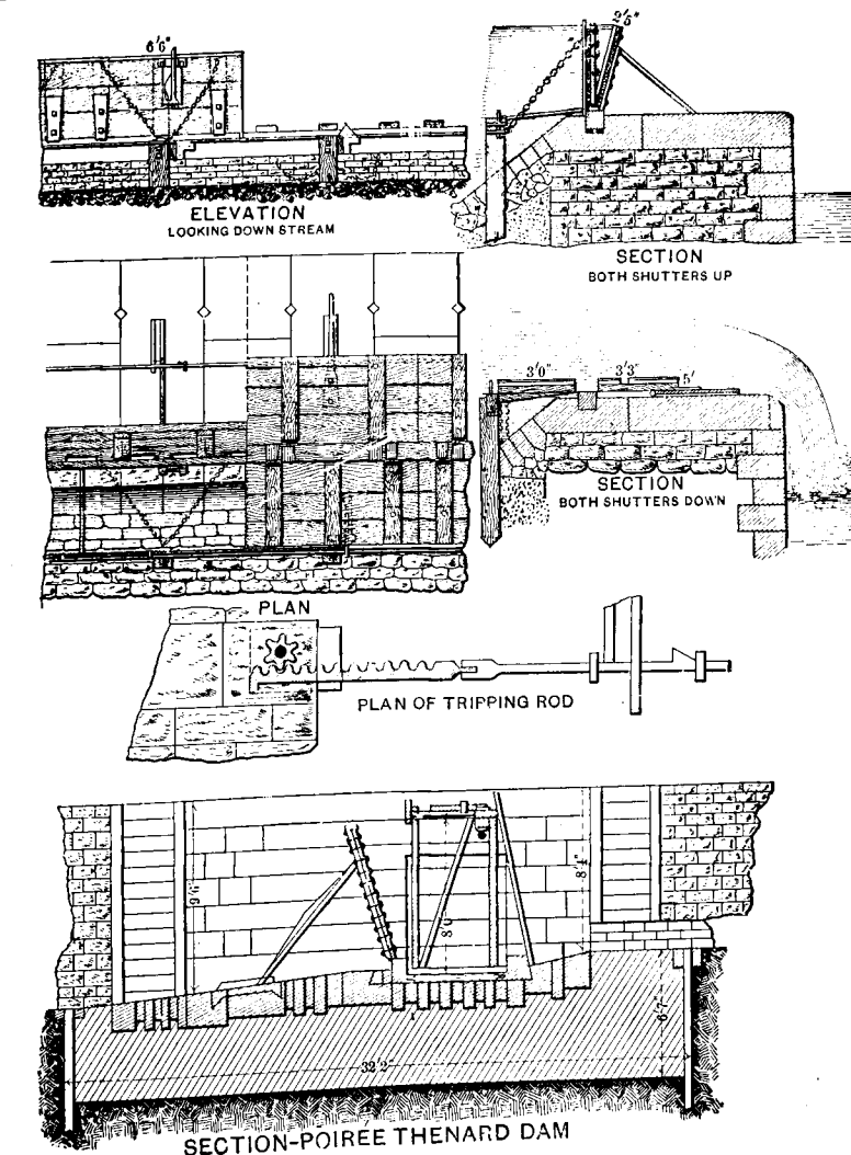
FIG. 226a.—Details of Thénard Dams.
