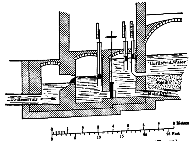
FIG. 6.—REGULATION APPARATUS AT BERLIN (TEGEL).
