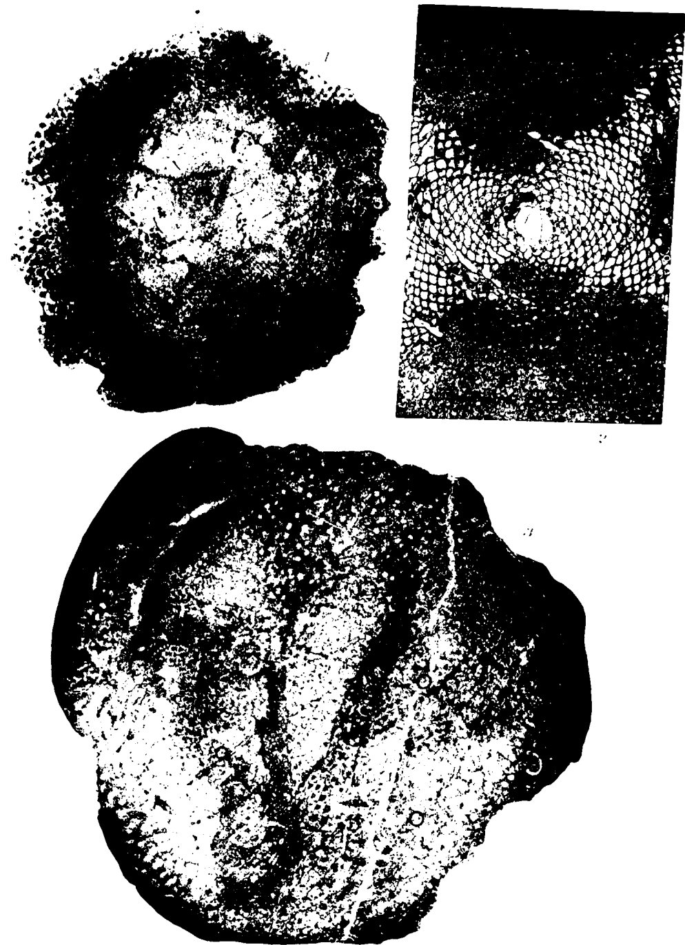
1. Orbitoides minor , Schlumberger. 2. Orbitoides media , d'Arnaud. 3. Orbitoides apiculata , Schlumberger.
