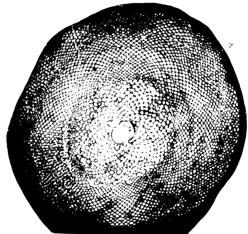
Orbitoides Hollandi n. sp.
