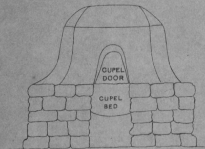
a. Front Elevation
