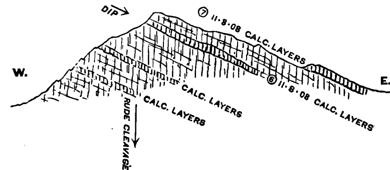
FIG. 1.—Muschelkalk spur N.N.E. of Khunmu.
