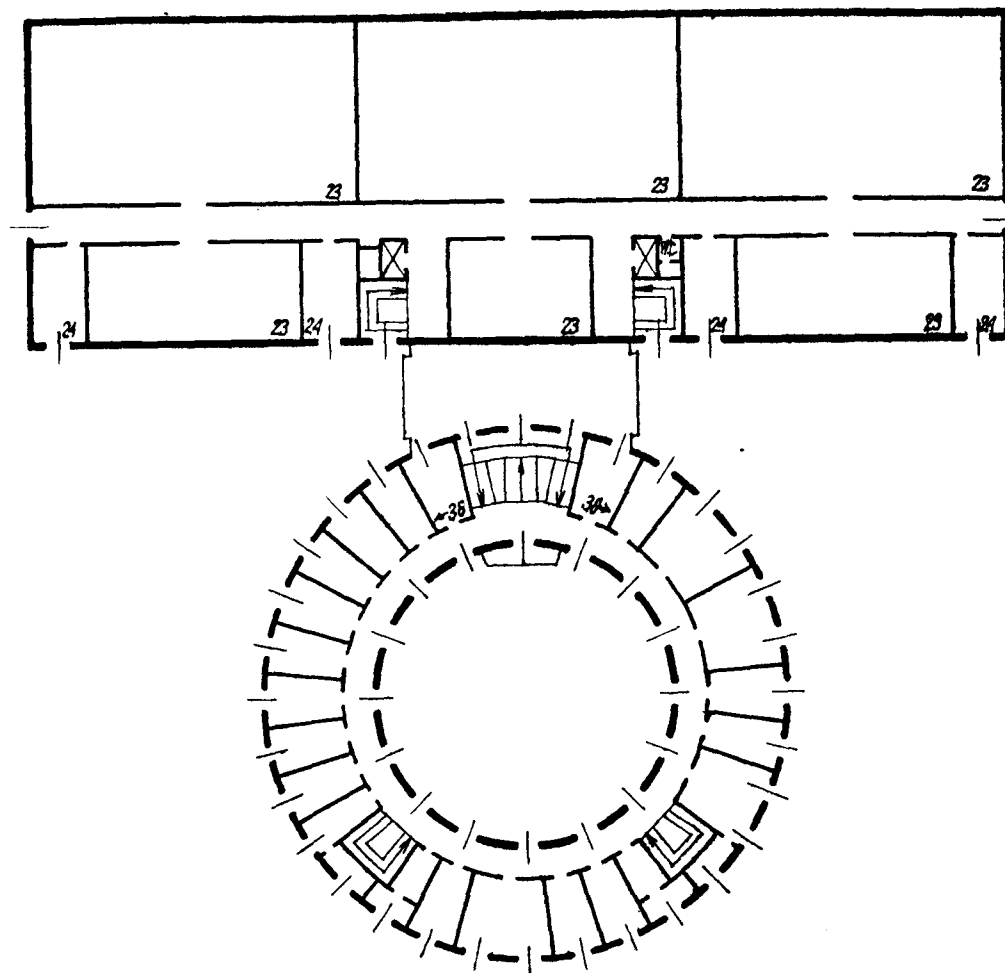
F. — Bâtiment central des Archives d'État, Varsovie (Plan du 3 e étage)
