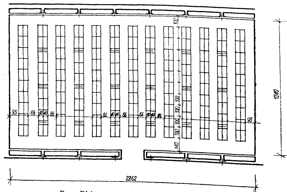
B. — Bâtiment central des Archives d'État, Varsovie (Système de rayonnages dans une section de dépôt)
