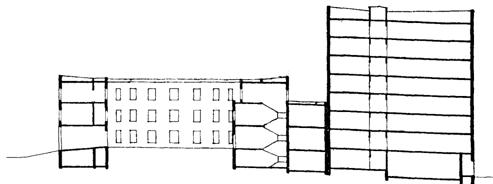
A. — Bâtiment central des Archives d'État, Varsovie (Coupe dans l'axe du bâtiment)
