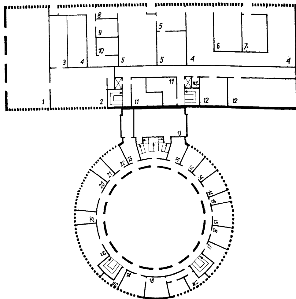
C. — Bâtiment central des Archives d'État, Varsovie (Plan du rez-de-chaussée)
