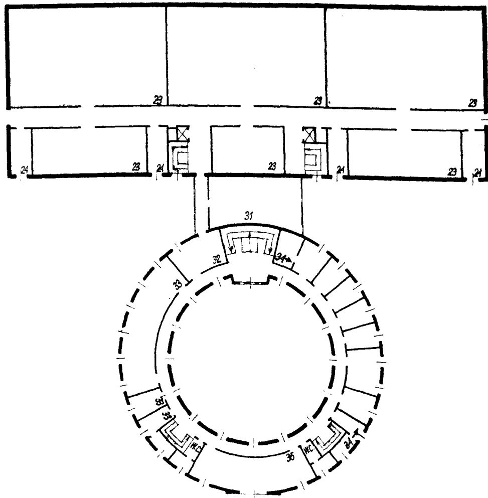
E. — Bâtiment central des Archives d'État, Varsovie (Plan du 2 e étage)
