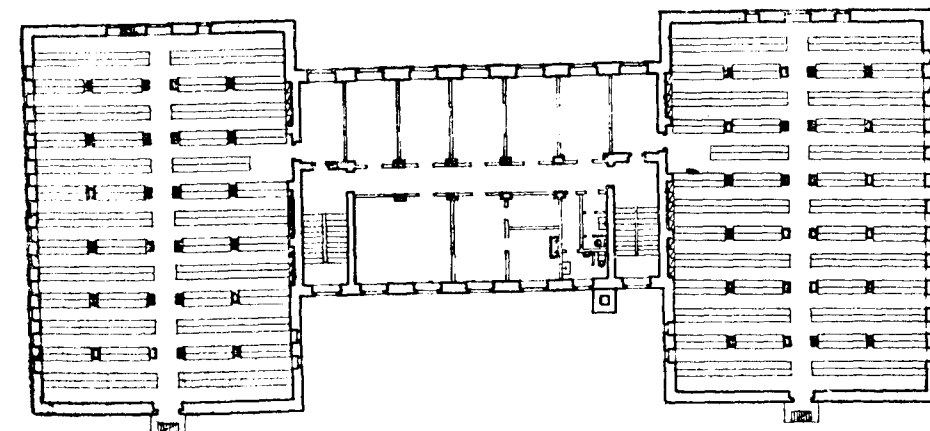
Projet-type d'un bâtiment d'une capacité de 1 200 000 articles (Plan du 2 e étage)
